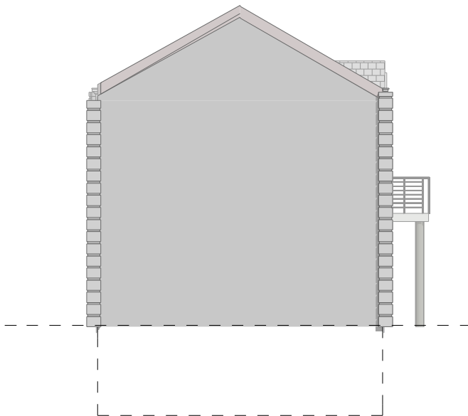
M.Mme Carlos LOPES PIGNON GAUCHE CHELLE 1/100
